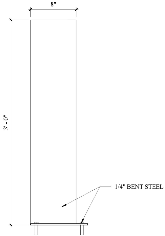
ELEVATION
